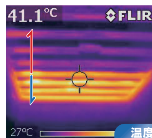
ルーフパネル裏面の状況 (サーモグラフィー)
